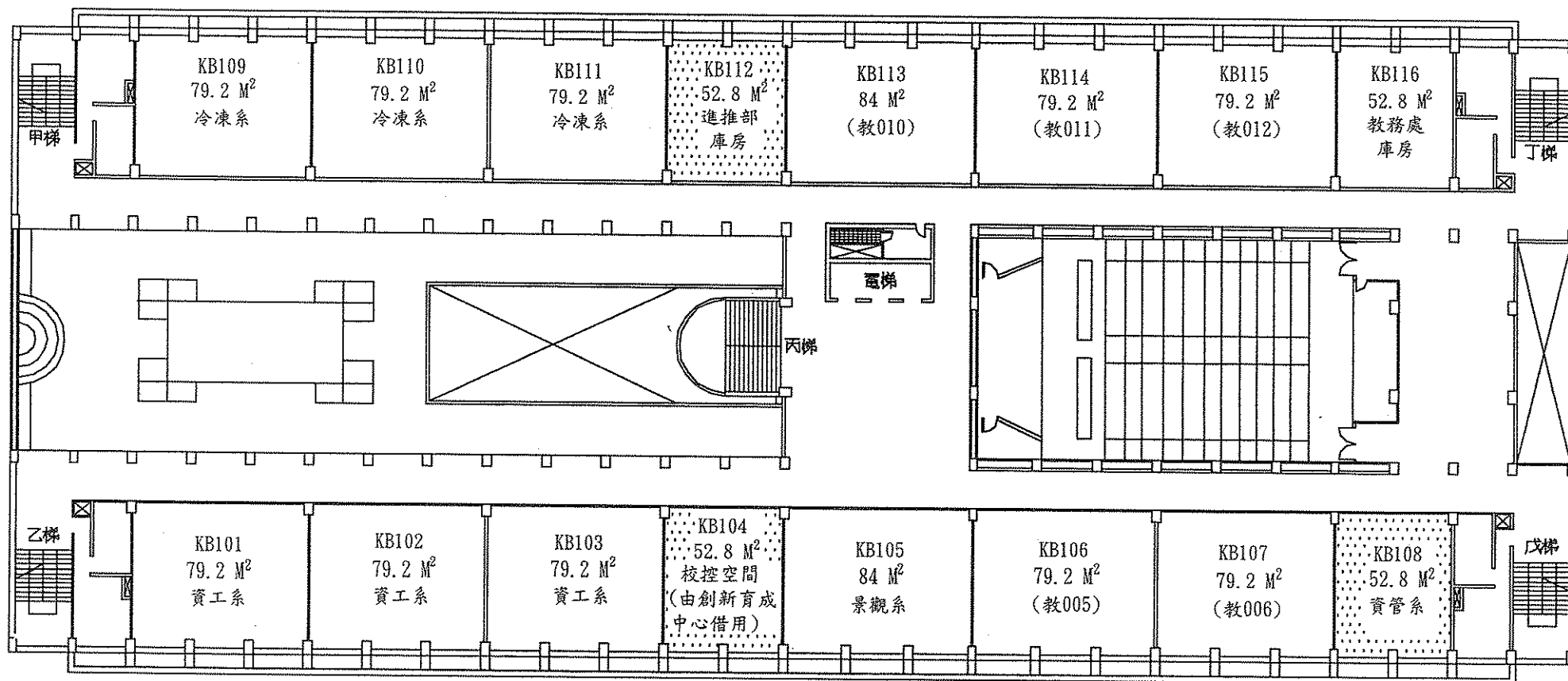
國秀樓地下一樓
